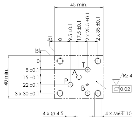
Anschlusslochbild 4/2-Wegesitzventile
