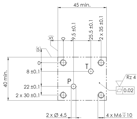
Anschlusslochbild 4/2-Wegesitzventile
